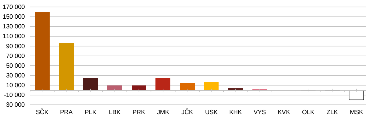
Graf 6 Srovnání krajů dle migračního přírůstku v letech od 2000 - 2011
