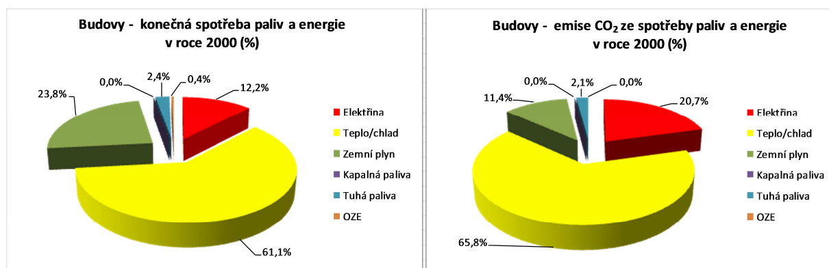
Obrázek 27: Spotřeba paliv a energie a emise CO 2 v sektoru budov v roce 2000 (výchozí bilance v členění dle druhu paliv a energie)
