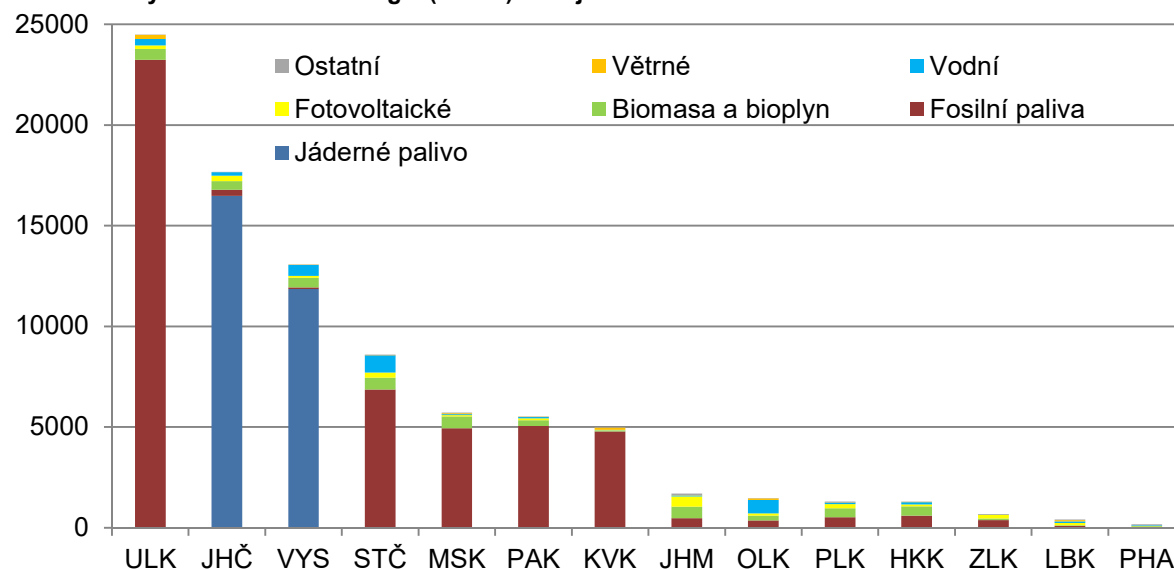
Obr. 5.1.1: Výroba elektrické energie (brutto) v krajích ČR v roce 2017
