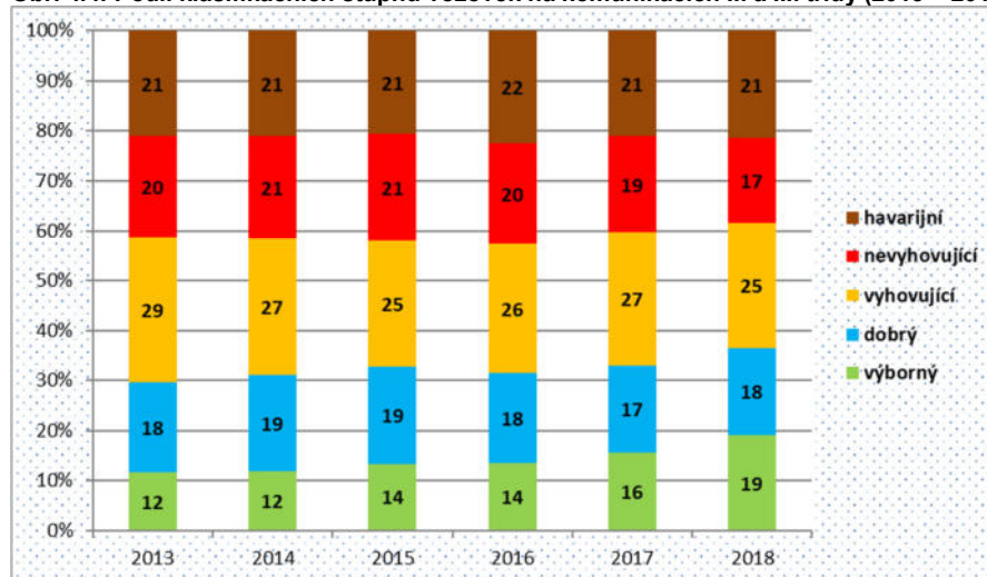
Obr. 4.4: Podíl klasifikačních stupňů vozovek na komunikacích II. a III. třídy (2013 – 2018)
