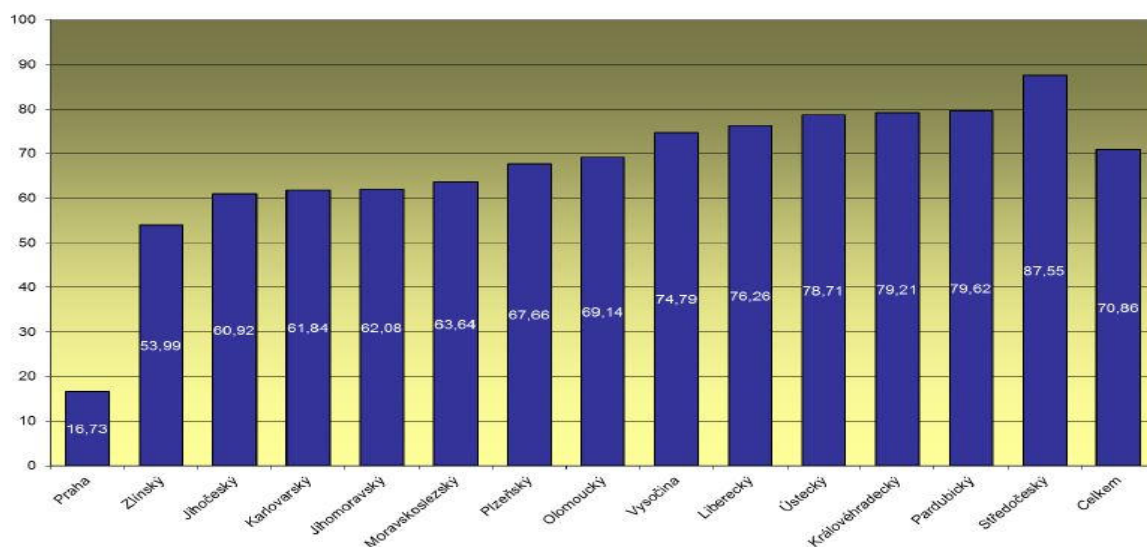
Obr. 4.2: Hustota silniční sítě v ČR podle krajů (km silnic na km 2 ) v roce 2017
