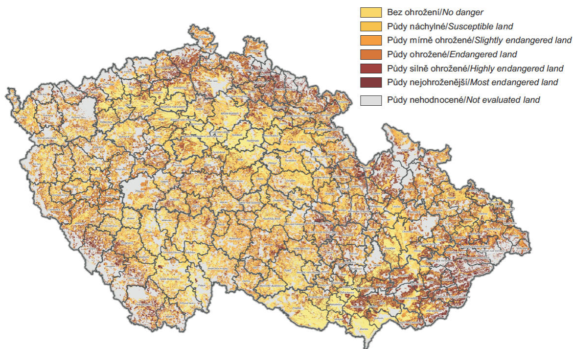
Obr. 9.2: Potenciální ohrožení zemědělských půd vodní erozí na území ČR
