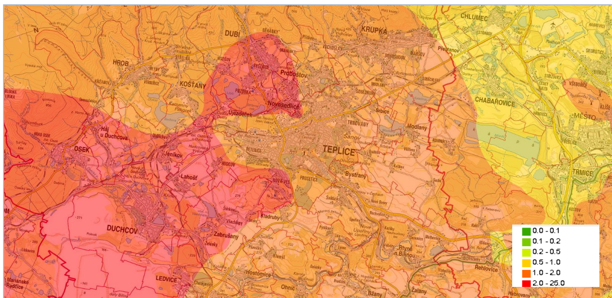
Obrázek 13 Mapa znečištění emisemi SO_2 ( \mu g/m^3 )
