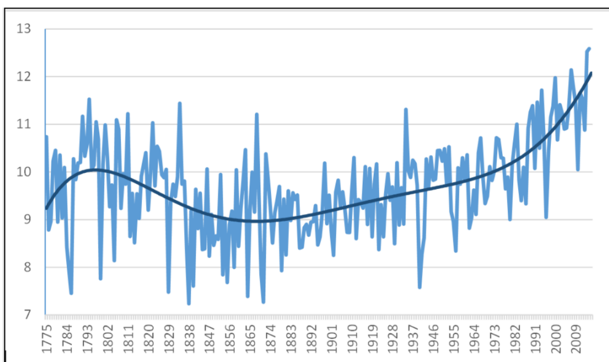
Obr. 1: Průměrné roční teploty vzduchu (v ^{\circ}\text{C} ) v období 1775–2015 na meteorologické stanici Praha-Klementinum. (Zdroj: ČHMÚ, 2016, portal.chmi.cz a infomet.cz .)
