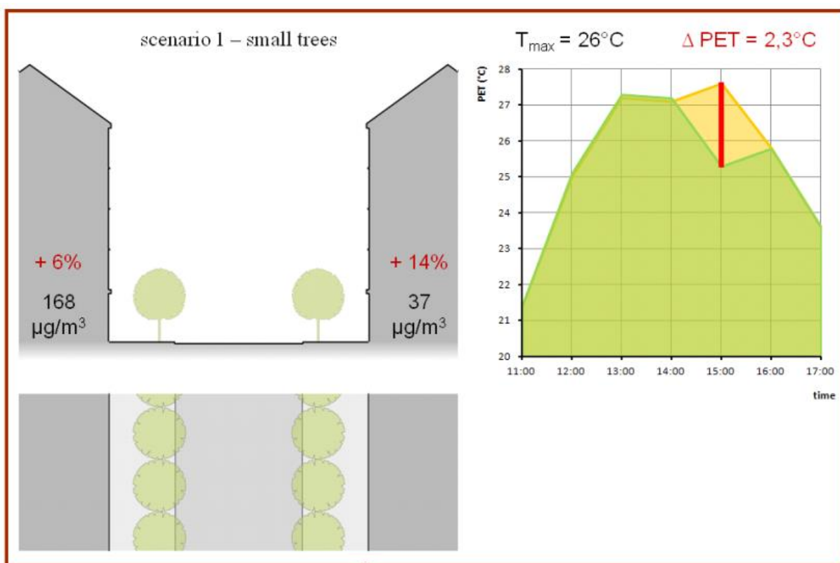
Obr. 5: Výstupy z modelování teploty a koncentrací škodlivin v Legerově ulici.
