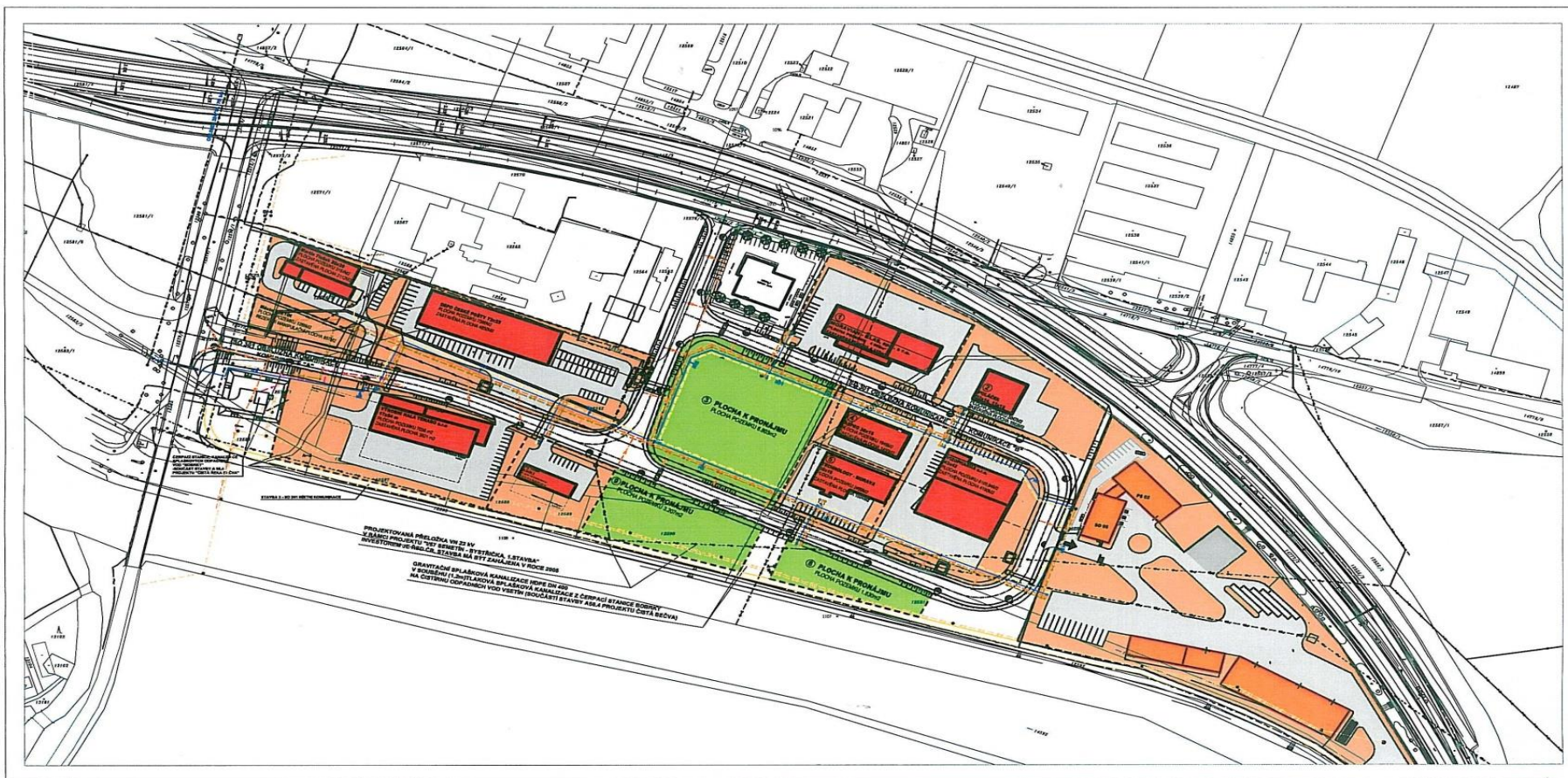
PRŮMYŠLOVÁ ZÓNA VSETÍN, BOBRKY II CELKOVÁ SITUACE M 1:2000
