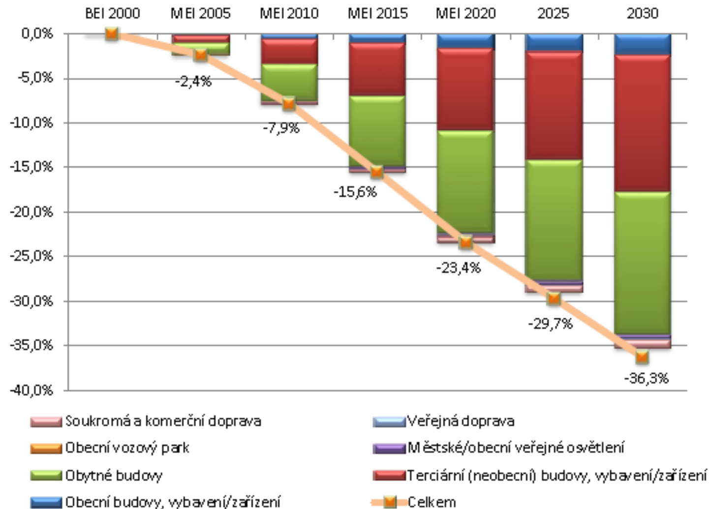
Graf 3 Odhad úspor emisí CO 2 dle sledovaných sektorů ve výhledu do roku 2030
